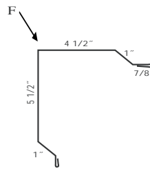
Ⓒ 29 Ga. Gable Trim 10'2" TLGT5xx
