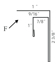
Ⓛ 29 Ga. "F" & "J" 10'2" TLFJ12xx
