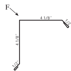
Ⓓ 29 Ga. AG4 Gable Trim 10'2" TLFS17xx
