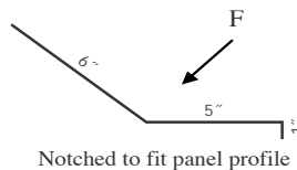
Ⓚ 29 Ga. Notched Endwall EL 42" TLNEEL32xx
