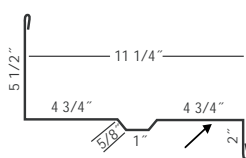
Ⓛ 29 Ga. 11.25" Fascia & Soffit 10'2" TLFS17xx
