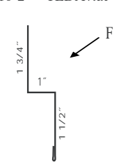
Ⓖ 29 Ga. Double Angle 10'2" TLDA7xx
