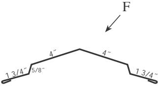
Ⓐ 29 Ga. 13" Univ. Ridge 10'6" TLURC1xx
