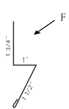
Ⓔ 29 Ga. Base Angle 10'2" TLBA3xx
