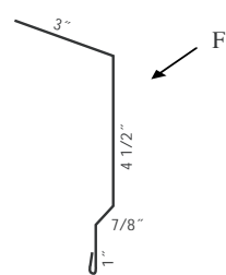
Ⓔ 29 Ga. Fascia Trim 10'2" TLFT4xx
