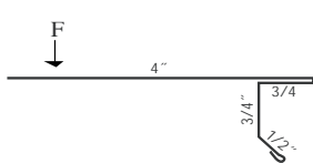
Ⓕ 29 Ga. Drip Edge 10'2" TL6.5F60xx
