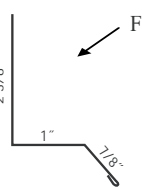
Ⓛ 29 Ga. 11.25" Fascia & Soffit 10'2" TLFS17xx
