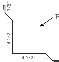
Ⓜ 29 Ga. Inside Corner 10'2" TLIC13xx
