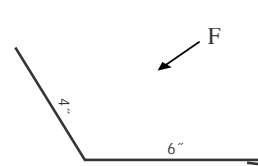
Ⓚ 29 Ga. Univ. Endwall 10'2" TLUE11xx
